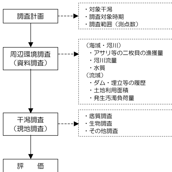
図 5-1 健全度評価の手順
